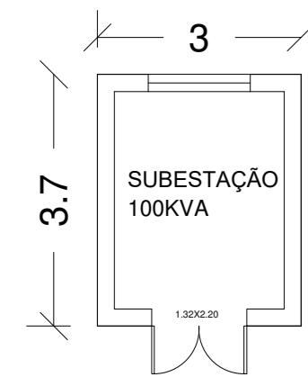
PLANTA BAIXA - SUBESTAÇÃO
